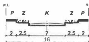
PRESJEK D-D
