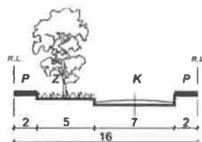
PRESJEK F-F
