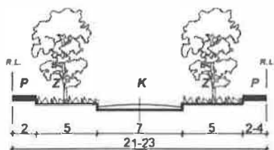
PRESJEK B-B
