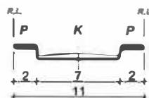
PRESJEK D-D
