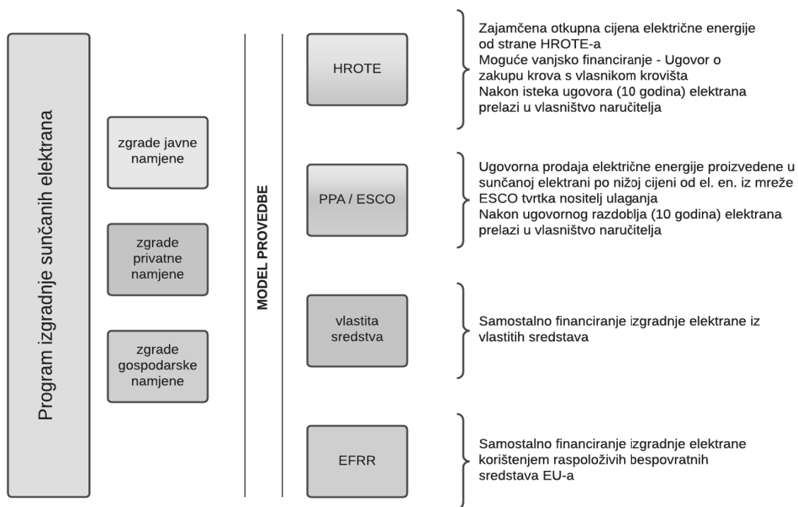
Slika 4.2. Pregled mogućeg modela izgradnje elektrane prema sektoru, odnosno vlasništvu
