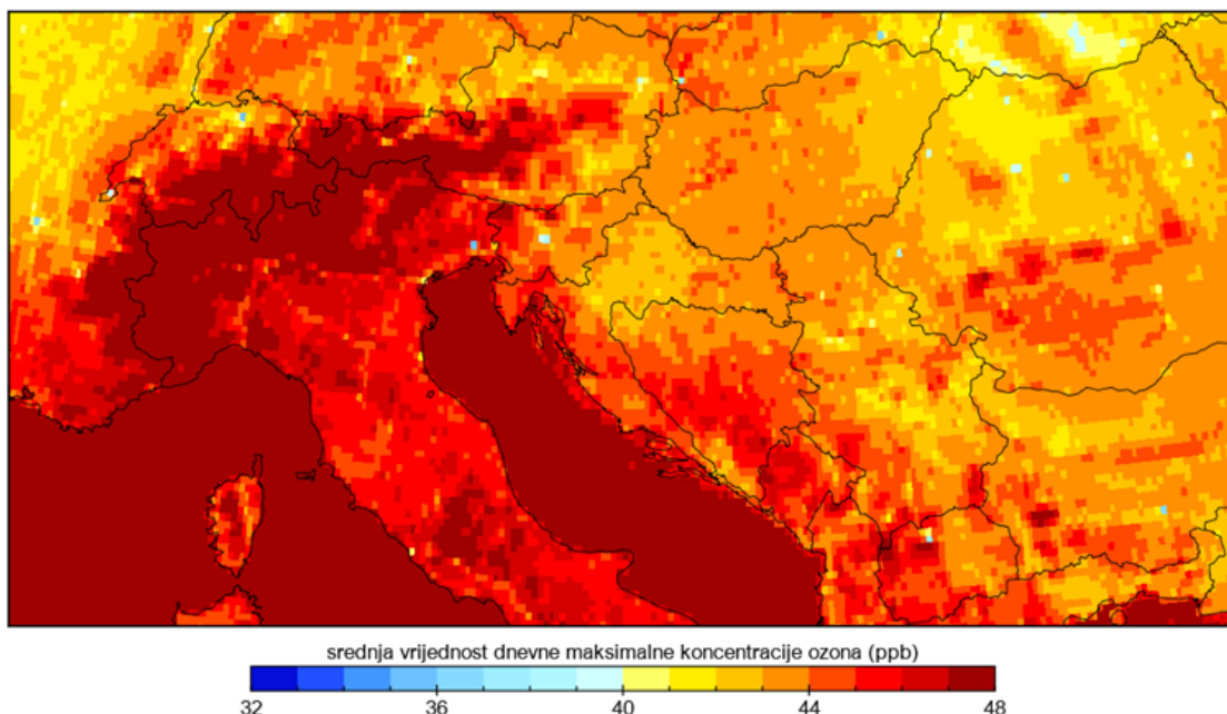
Sl. 3-1: Karta maksimalnih dnevnih koncentracija O_3 prema proračunu EMEP modelom za 2019. godinu na području Republike Hrvatske i širem okruženju
