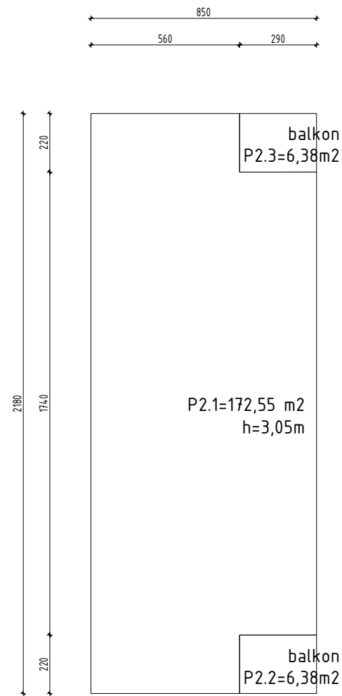
TLOCRT 2. KATA GBP=172,55m2
