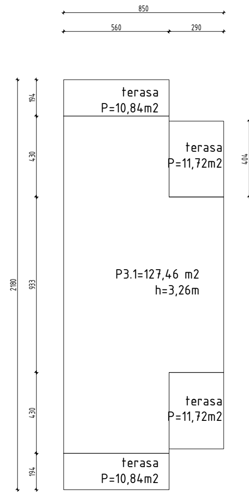
TLOCRT UVUČENOG KATA GBP=127,46m2
